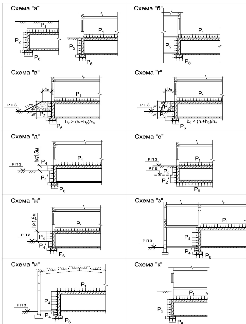
Рисунок 14.1 – Схеми прикладання приведених навантажень на конструкції захисних споруд та СПП
