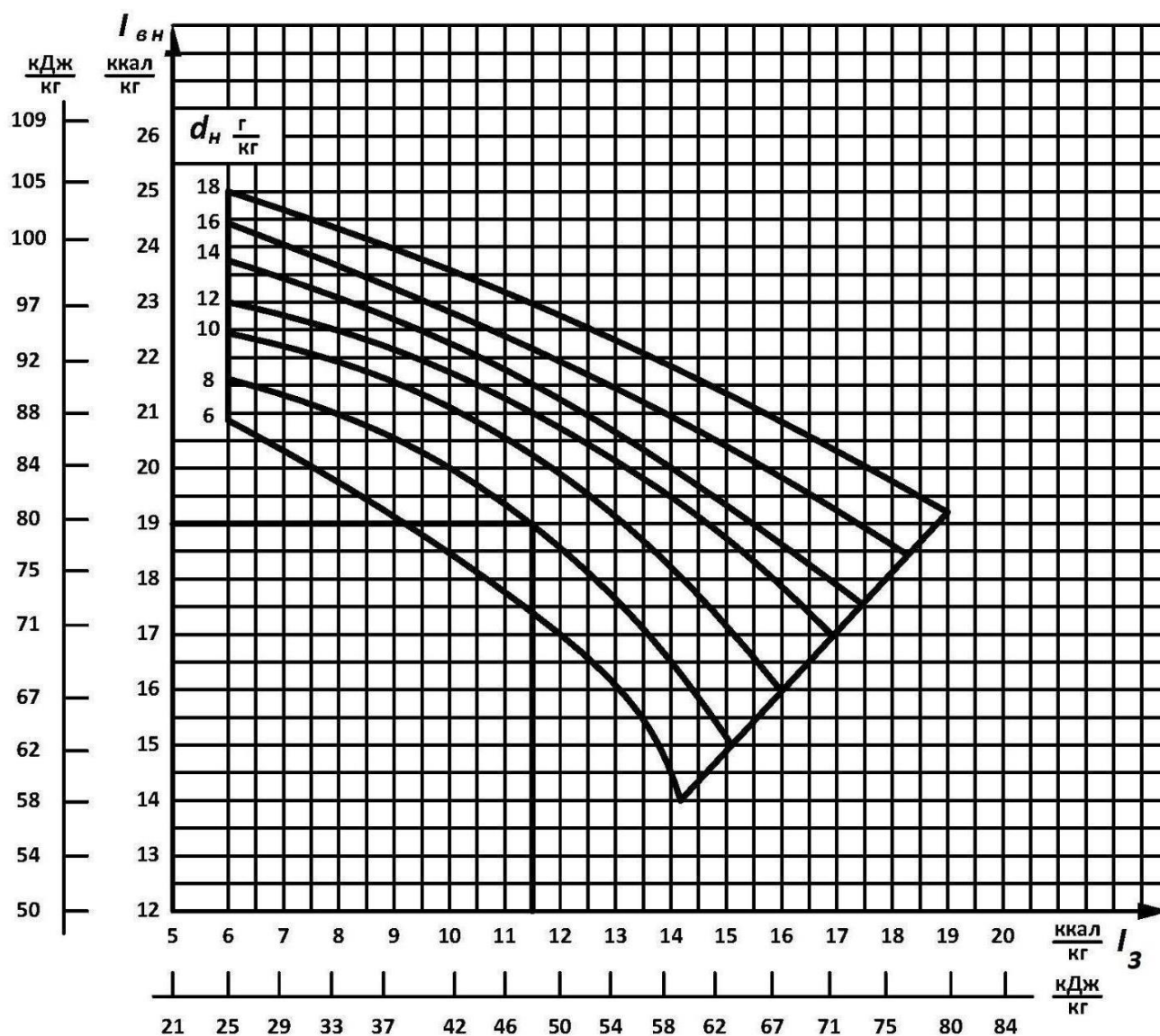
Рисунок Г.2 – Визначення тепловмісту (ентальпії) внутрішнього повітря при видаленні теплових надлишків системою вентиляції в I режимі (чиста вентиляція) та допустимих сполучень температури та вологості цього повітря для II і IV кліматичних районів
