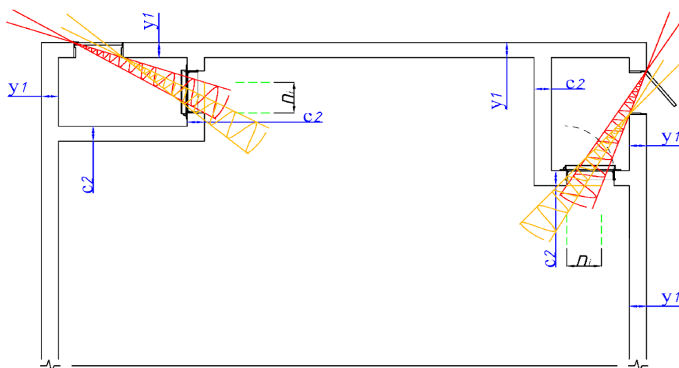
Рисунок Г.2.2 – Приклад умовного проникнення всередину захисної споруди радіоактивного випромінювання
